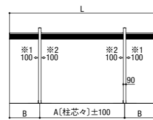
2台用 基本 (W:48~60型) 側面図
