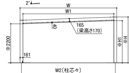
2台用 基本 正面図
