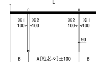
1台用 基本 (W:24~30型) 側面図
