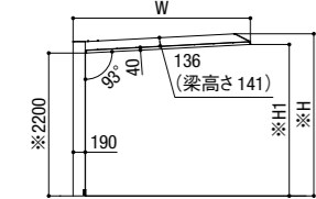
1台用 基本 正面図
