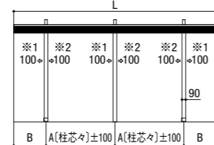
1台用 基本 (W:33型) 側面図
