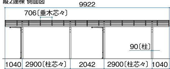
縦2連棟 側面図
