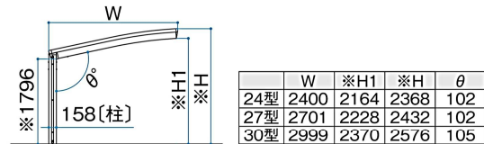
基本・縦2連棟 正面図
