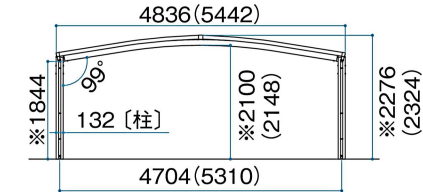
基本・縦2連棟 正面図
