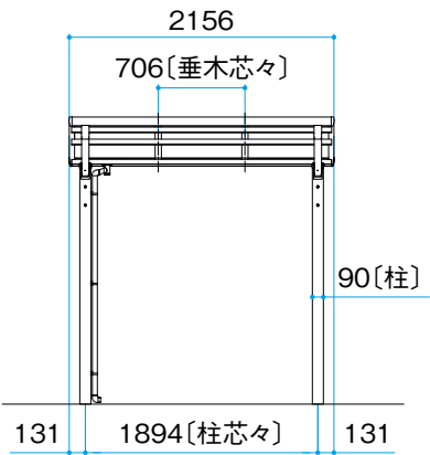
基本 側面図 L22
