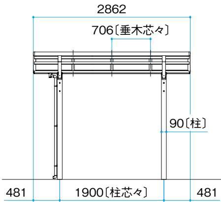
基本 側面図 L29
