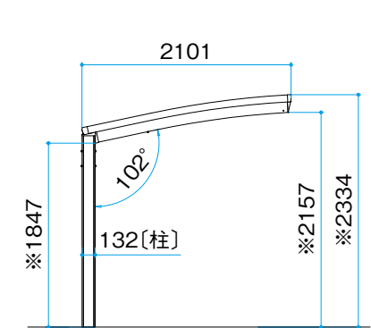
基本 正面図
