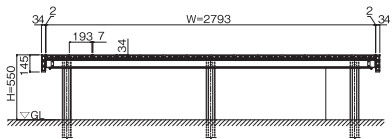
●1.5間 正面図
