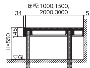
●1.5間、2.0間 側面図
