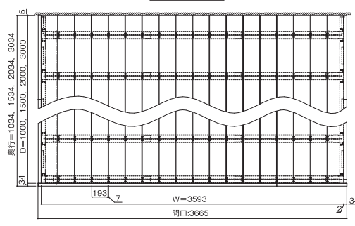
●2.0間 正面図
